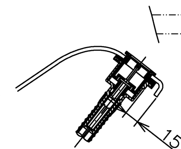
断面A-A(1:5)
