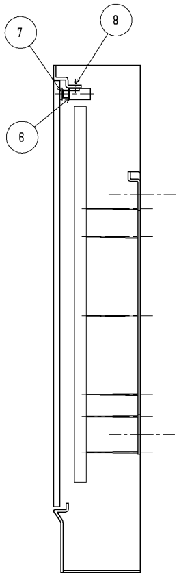
A-A断面図
