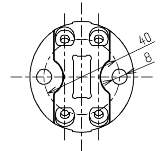
取付座詳細(1:2)
