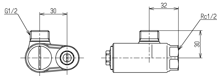
止水栓(2ヶ)
