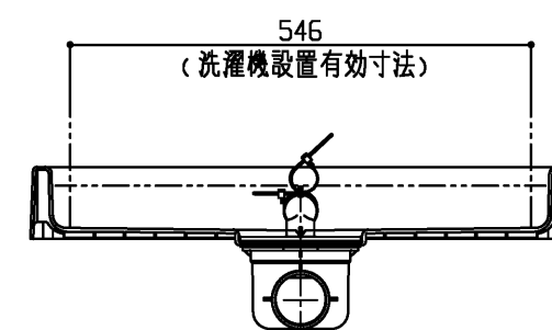
断面B-B
