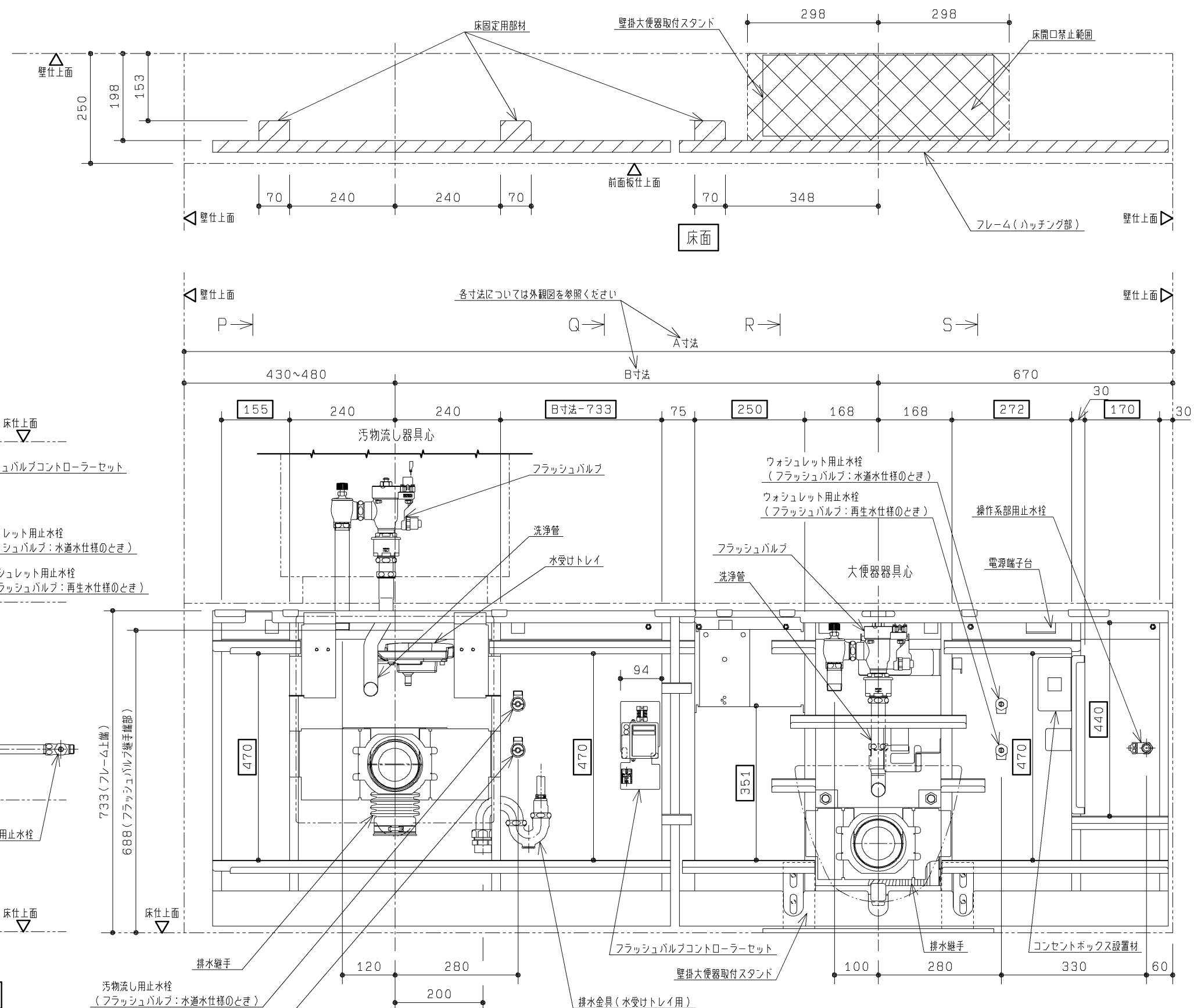
S 視図
