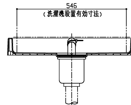
断面B-B
