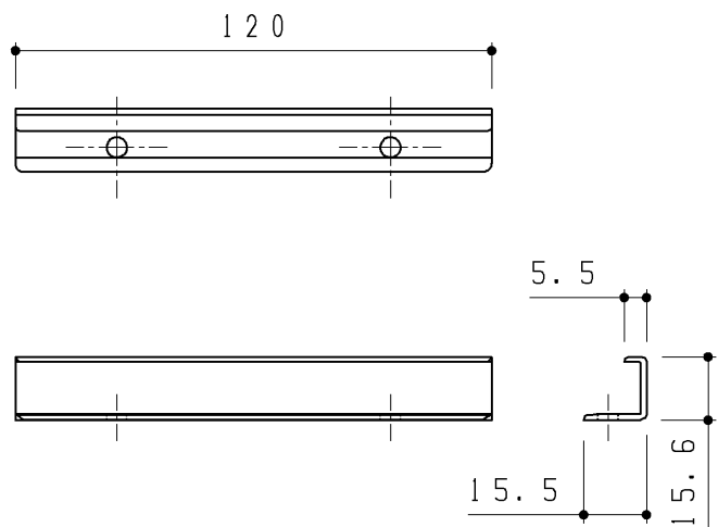
(S=1:5) 材質：PP
