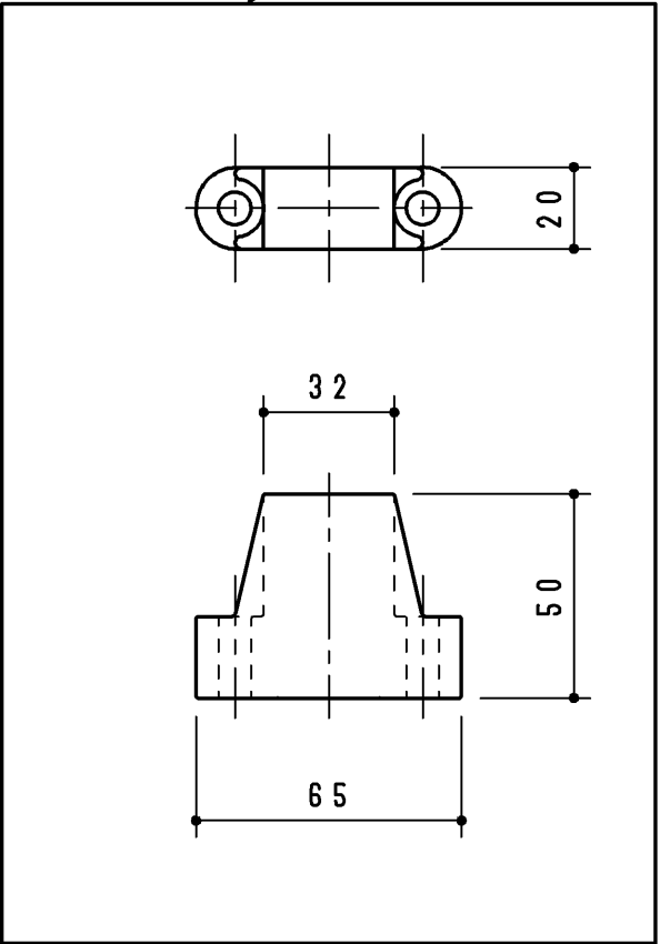
固定片 3ヶ所
