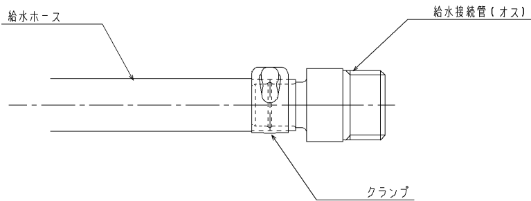
C部詳細図(S=1:1)
