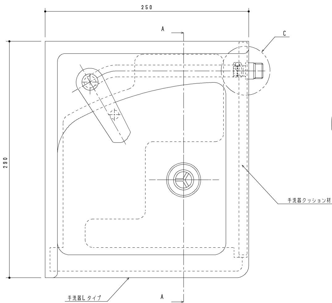
手洗器Lタイプ
