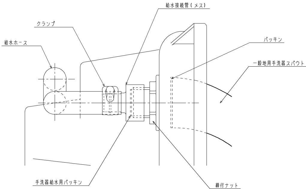
D部詳細図(S=1:1)
