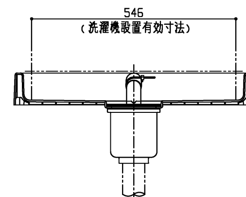
断面B-B
