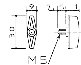
⑦ 固定ノブ (1:2)
