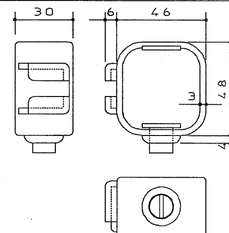
④ ハンガー (1:2)
