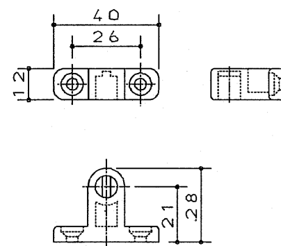
① バーホルダー (1:2)
