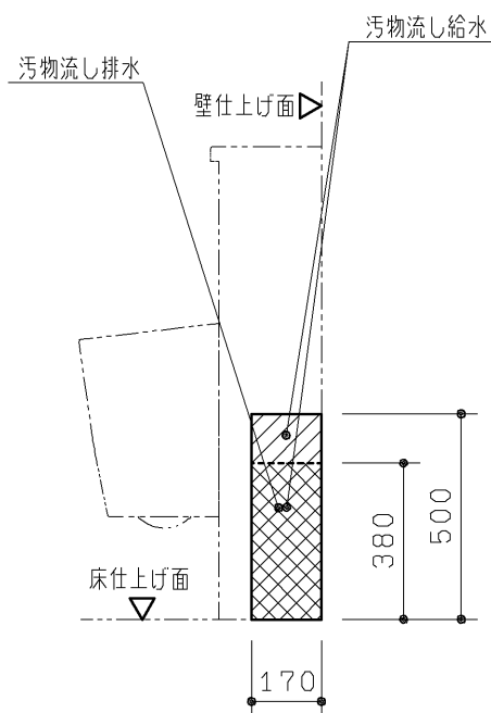
P 視図
