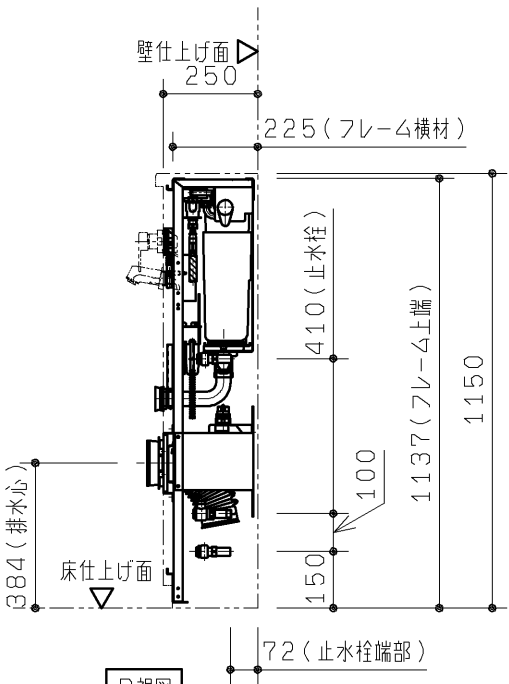
R 視図
