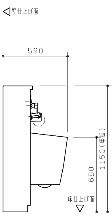
B矢視図
