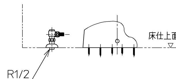
正面図
