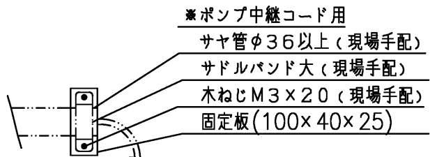
サイヤ管固定部詳細図
