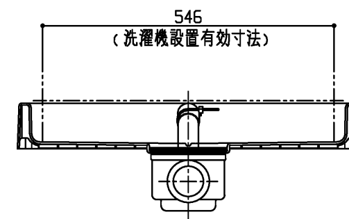
断面B-B
