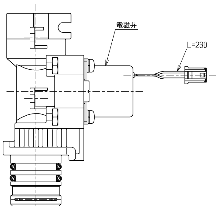
駆動部
