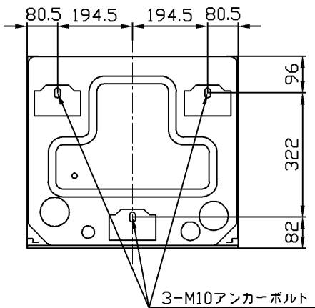
アンカーボルト位置 上面透視図
