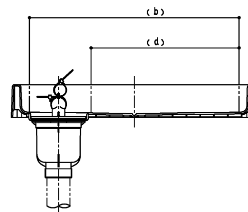
断面B-B
