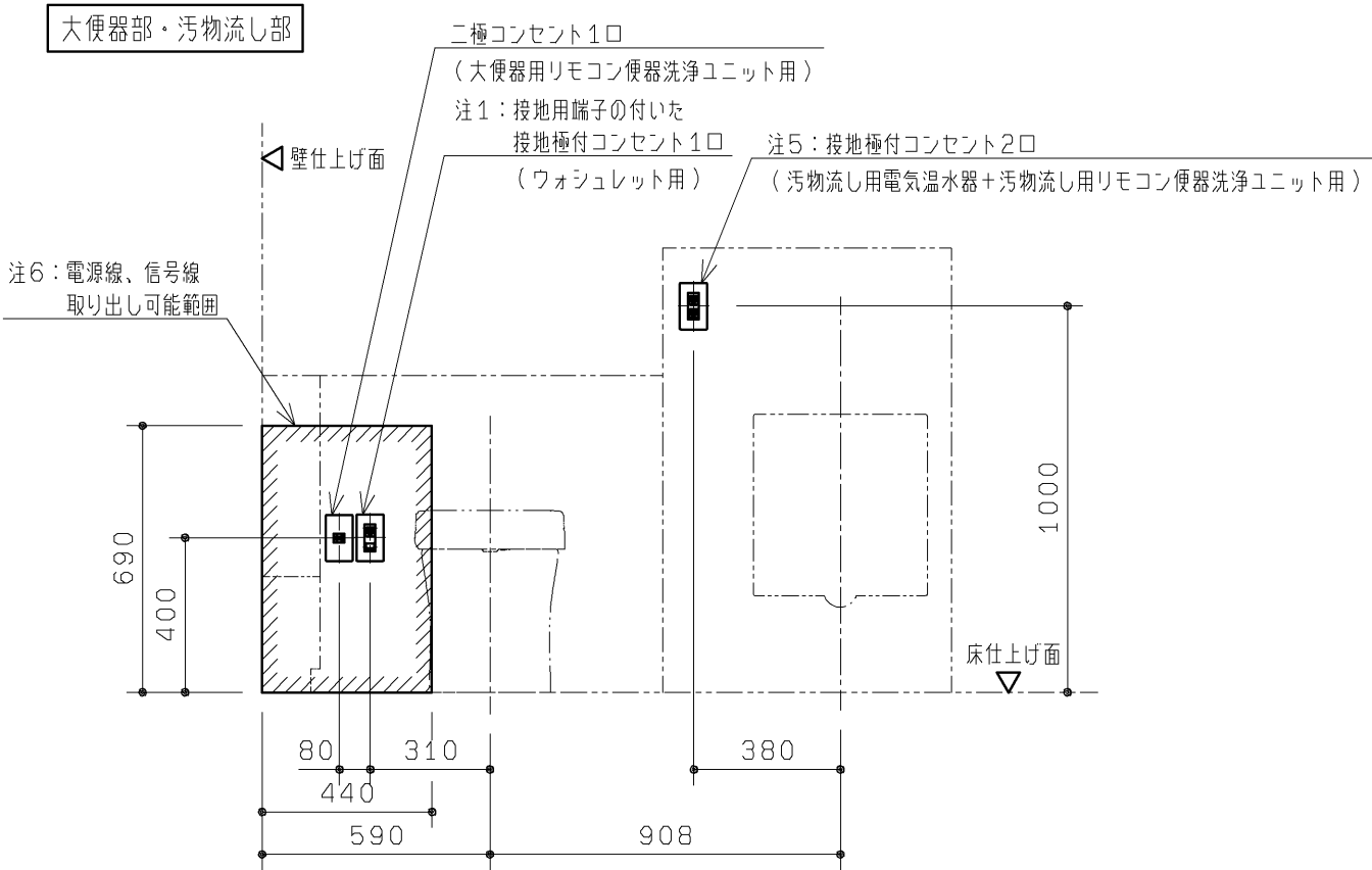
操作系部
