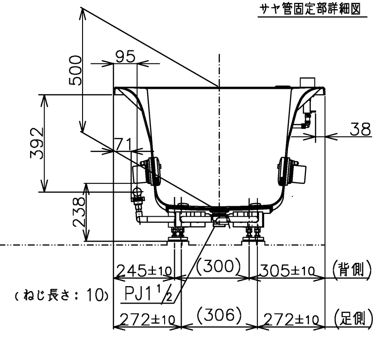
断面A-A
