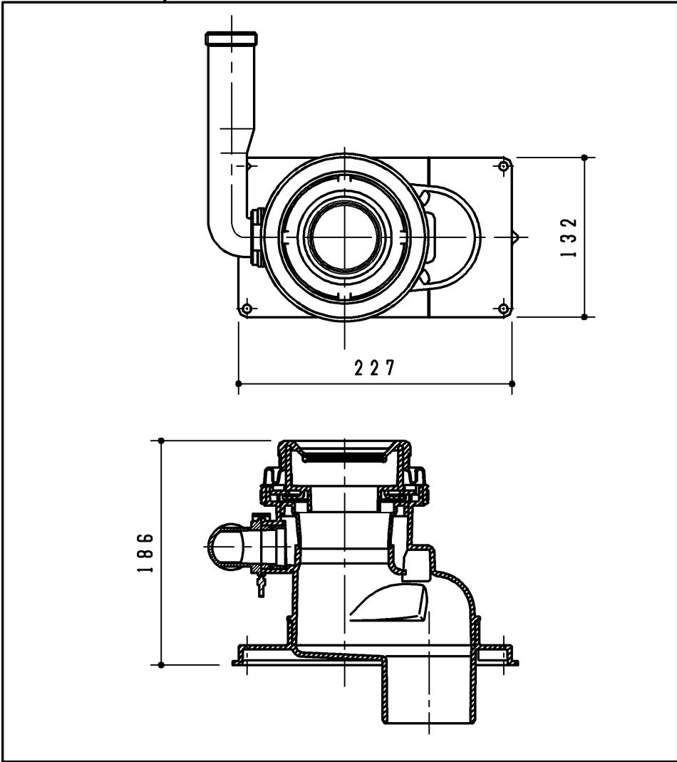
手洗排水管(間口調整用)
