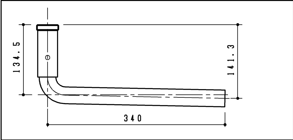
手洗排水管(間口調整用)
