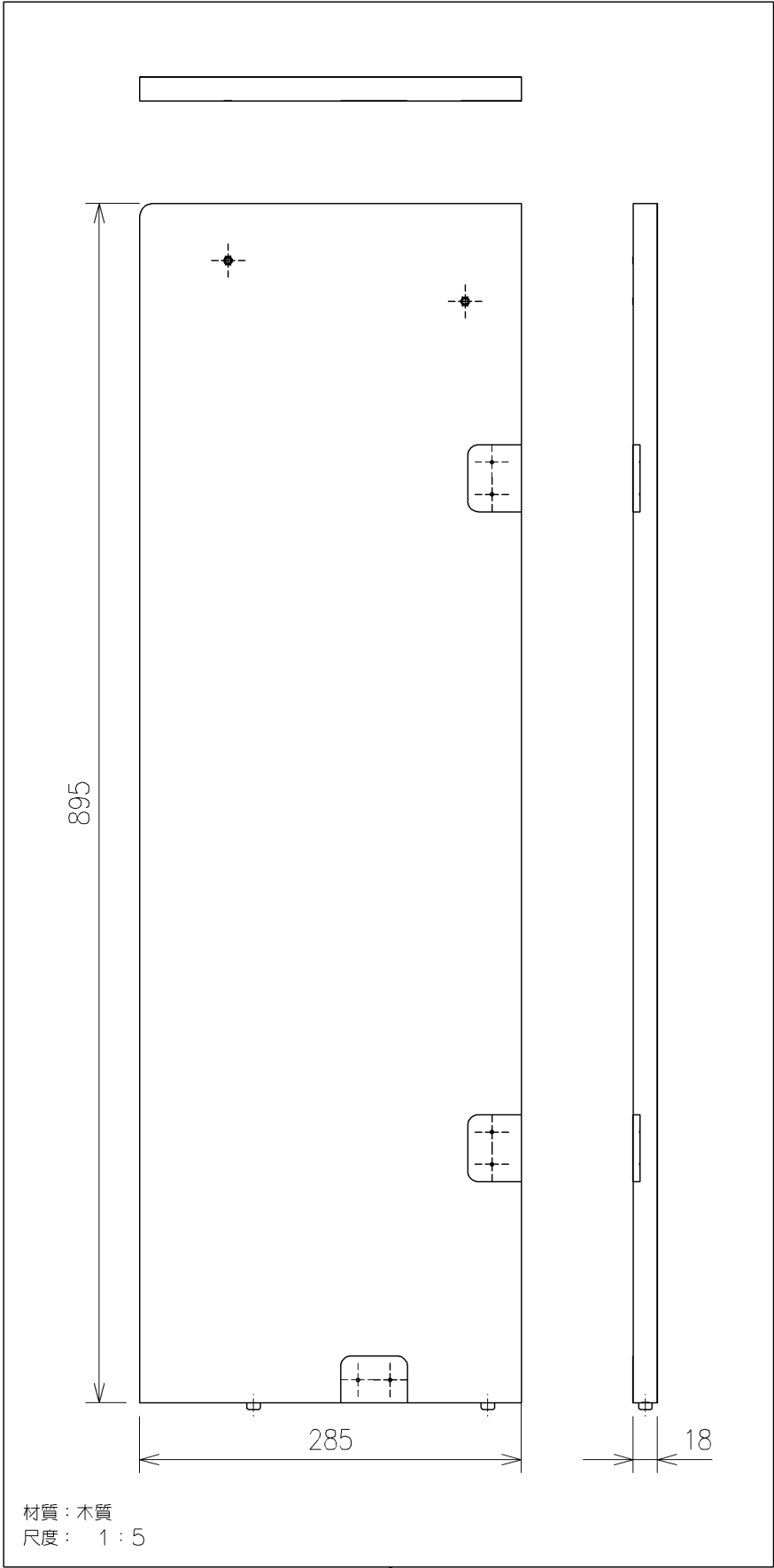
エンドパネル組品
