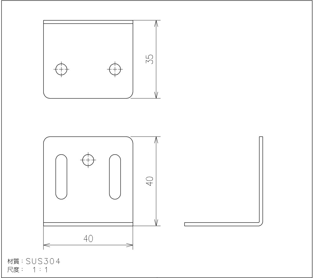
アングル材（3ヶ）
