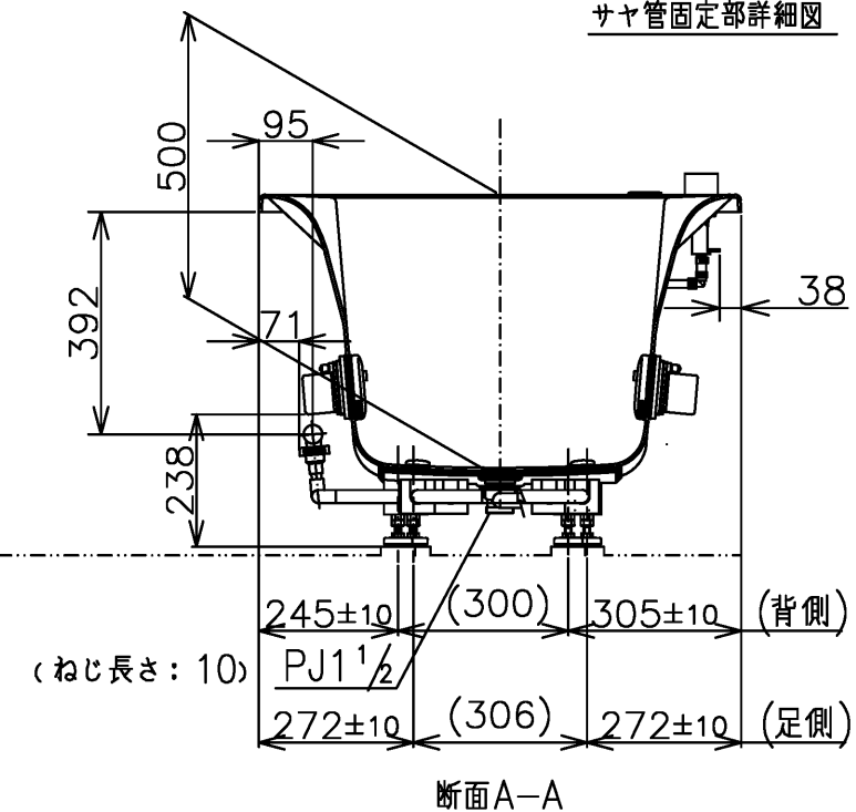
サヤ管固定部詳細図
