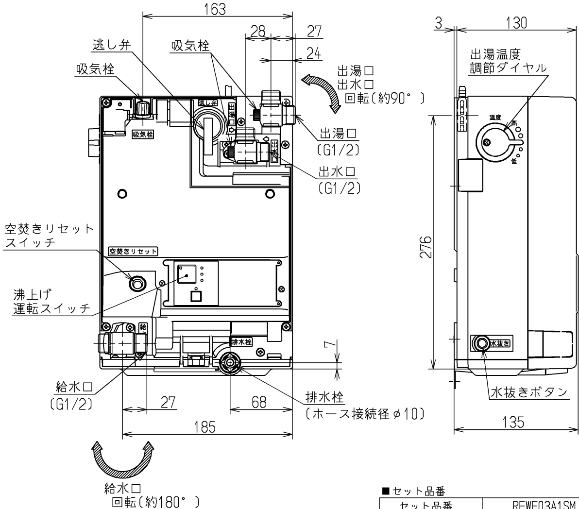
■化粧カバー取外図
