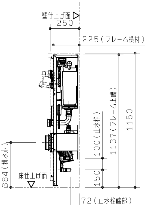
R 視図
