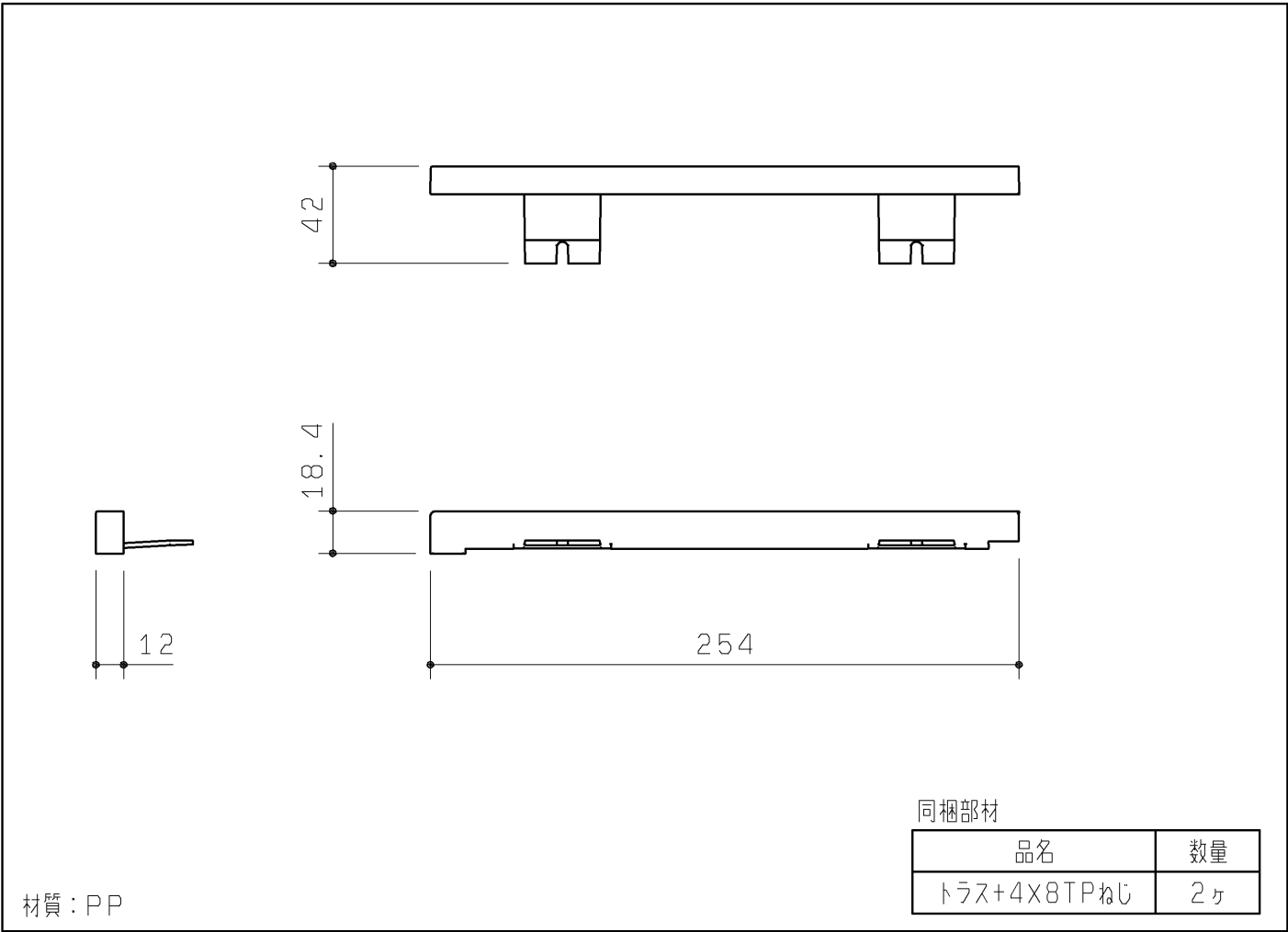
天板キャップセット ( L )
