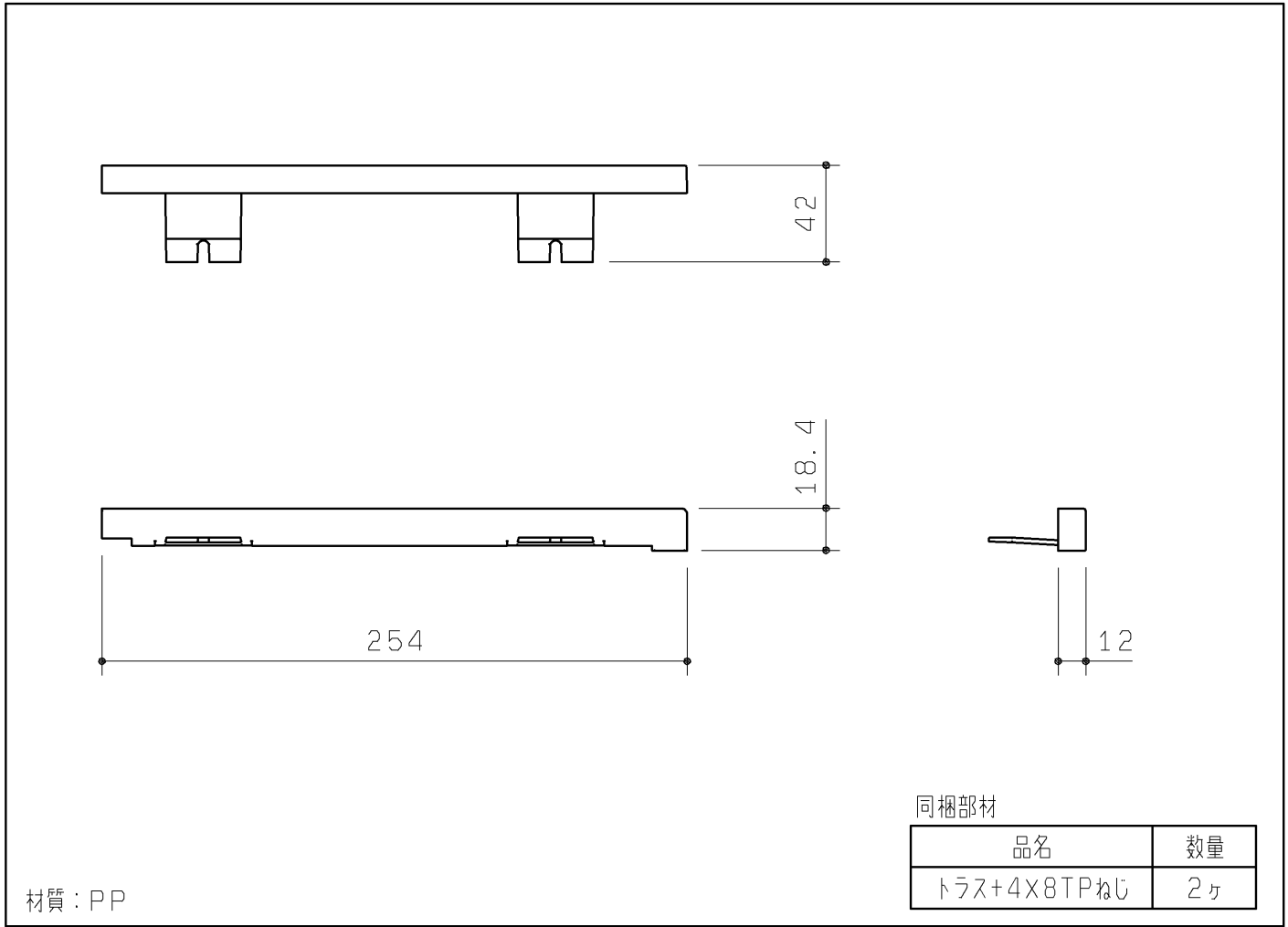
天板キャップセット ( R )
