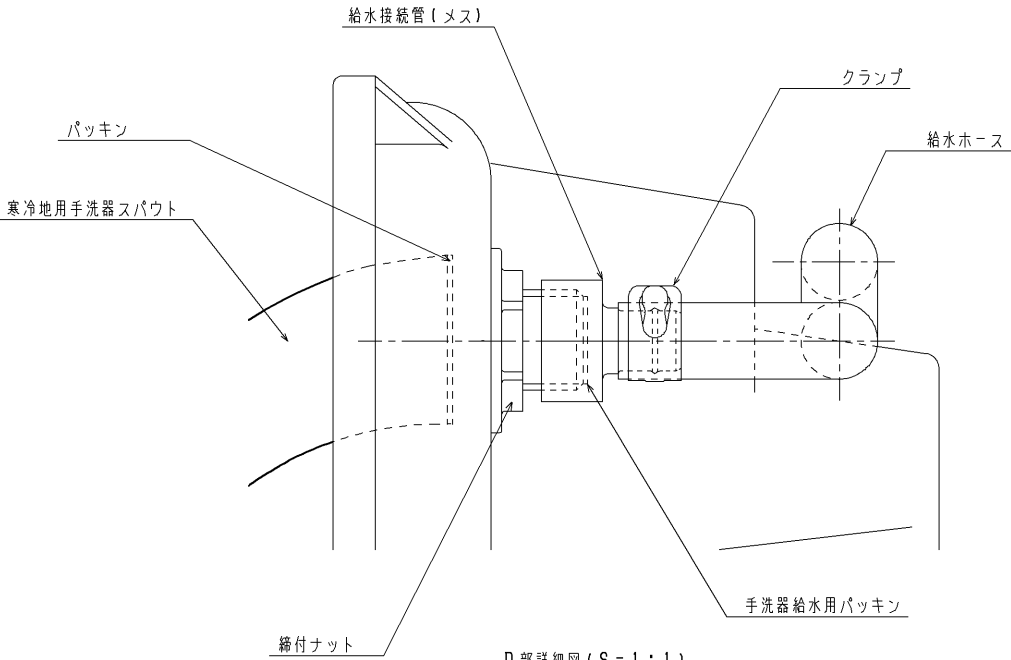
D部詳細図(S=1:1)
