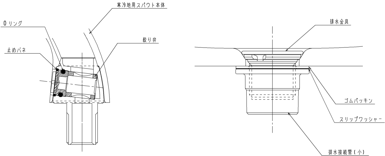
E-E断面詳細図(S=1:1)
