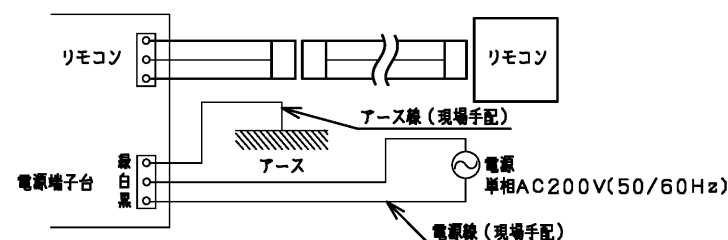
結線図
