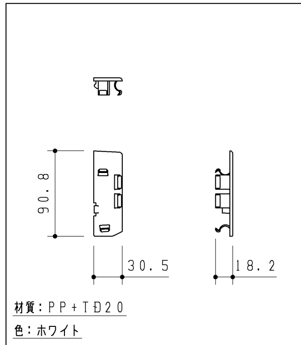
キャップ
