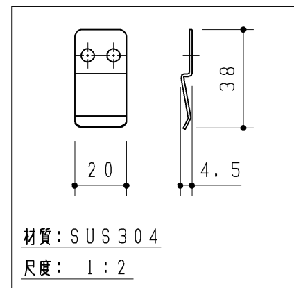
取付材 1ヶ
