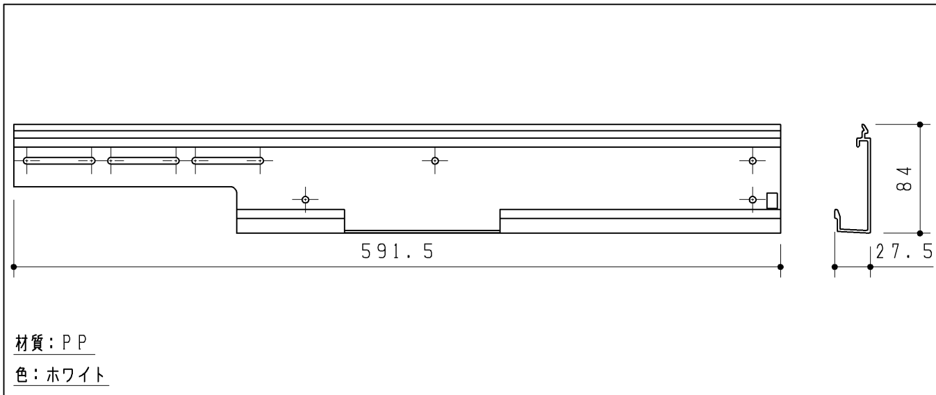
取付材
