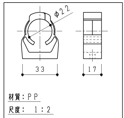
取付材 1ヶ
