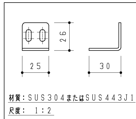
アングル 2ヶ
