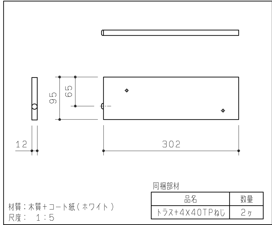
壁側板セット右
