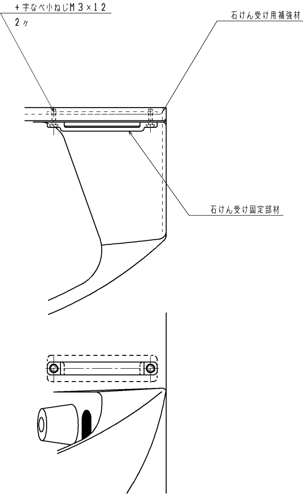
石けん受け固定部材取付け詳細 (S=1:2)
