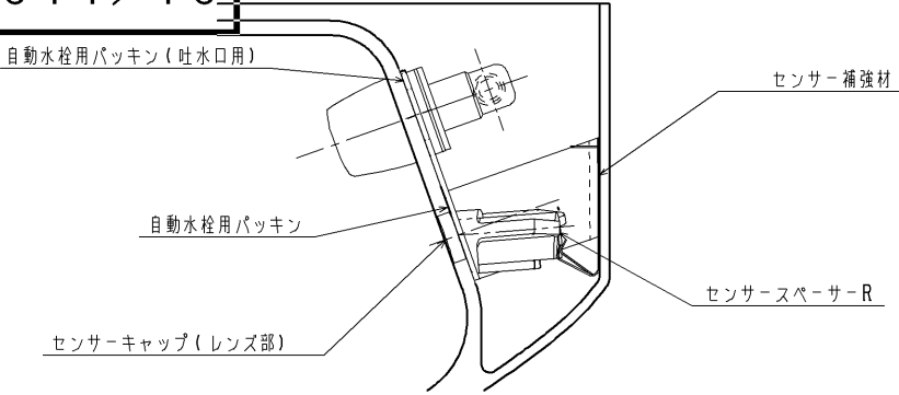
A部断面詳細図 (S=1:2)
