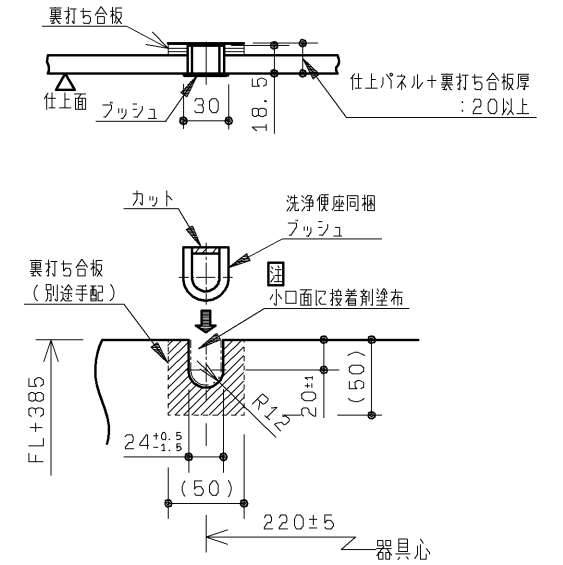
A部詳細図 (S=1:5)
