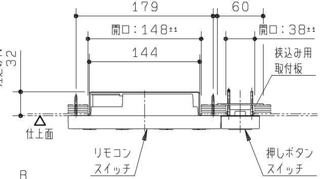
B-B断面詳細図 (S=1:5)
