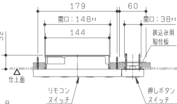
B-B断面詳細図（S=1:5）
