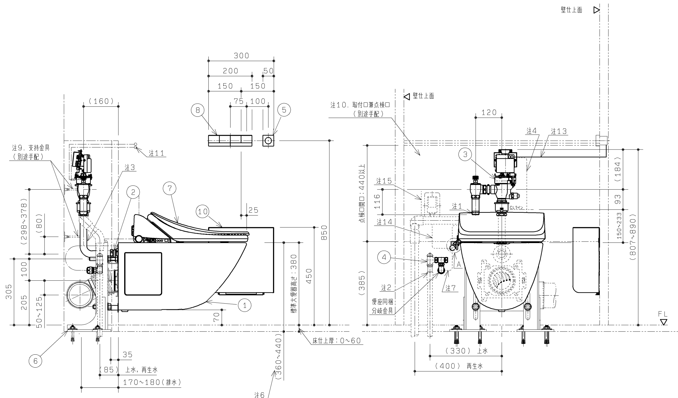
ウォシュレットホース, 電源コード, 信号線貫通部開口形状
