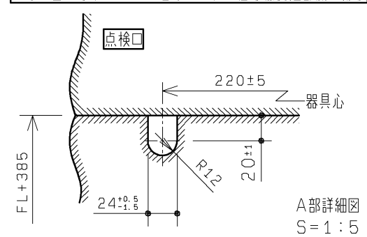
ウォシュレットホース, 電源コード, 信号線貫通部開口形状
