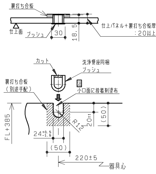
A部詳細図（S=1:5）
