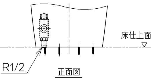
床給水仕様の場合
