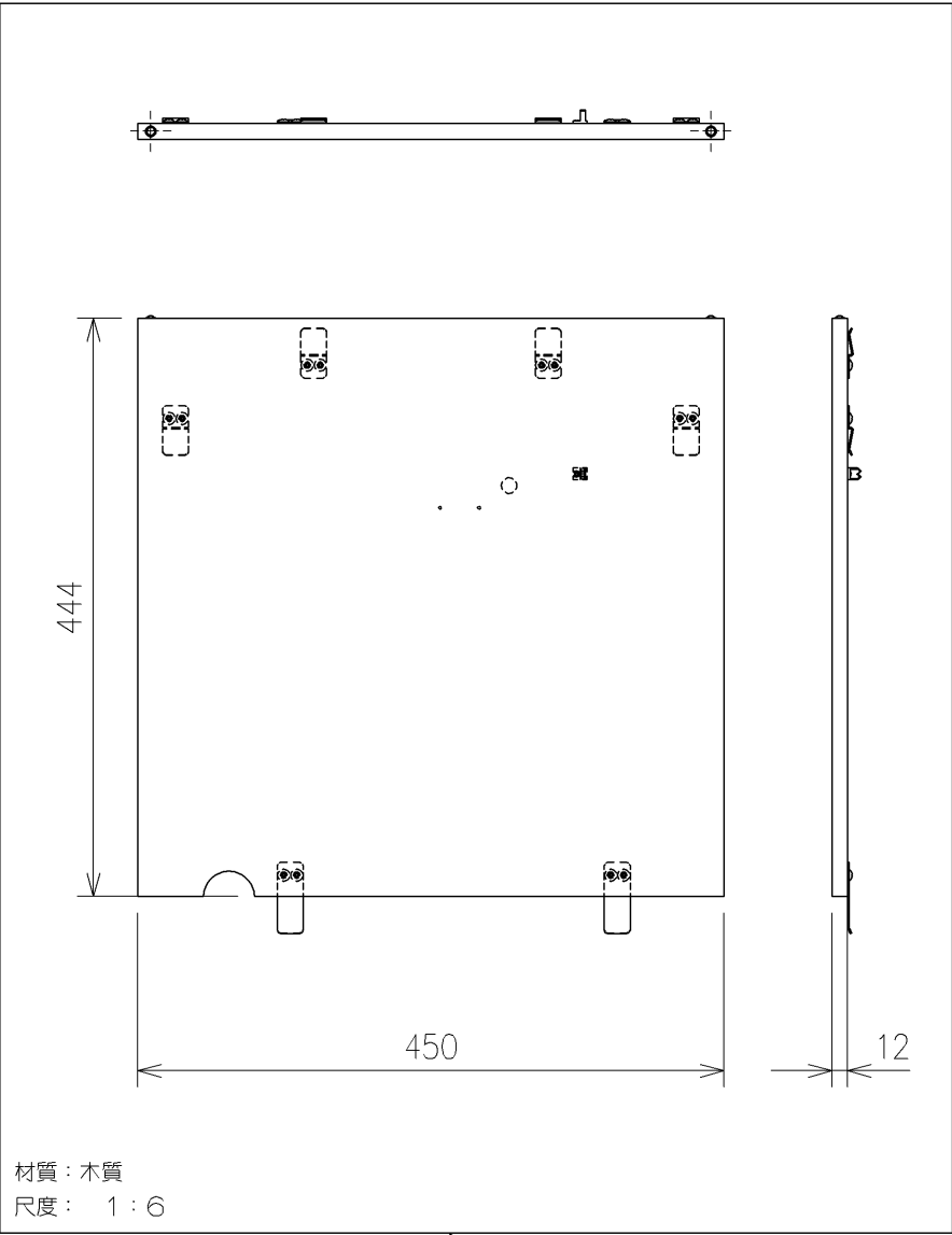
前板組品（照明）
