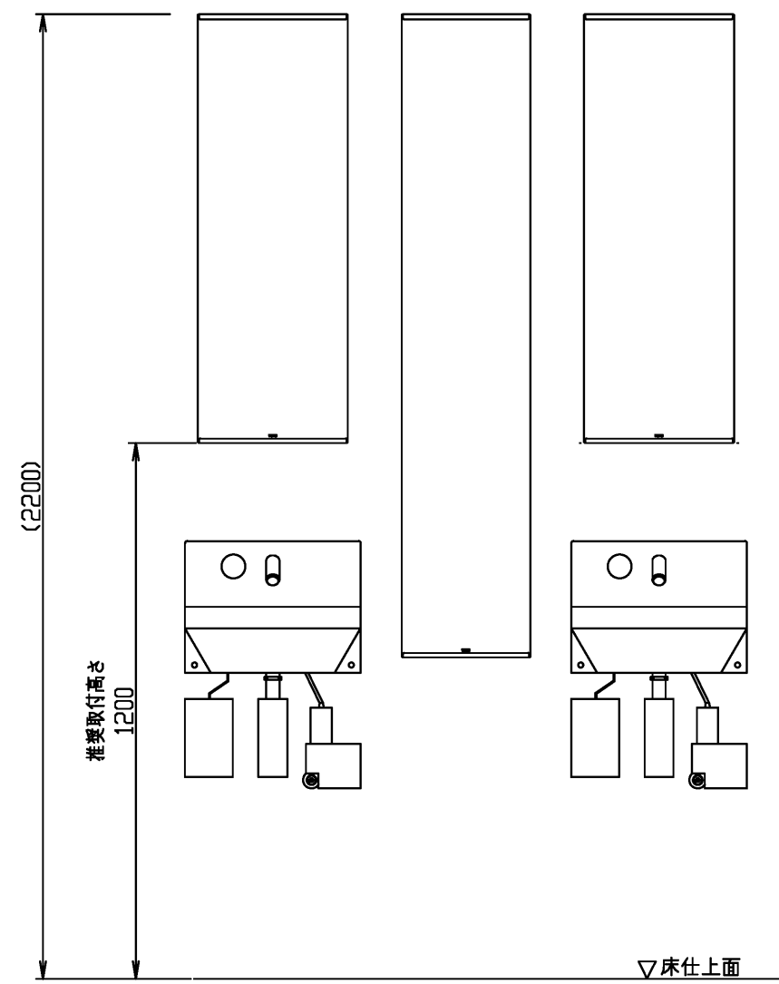
全身鏡・化粧鏡を併設したプランの取付高さ推奨取付位置
