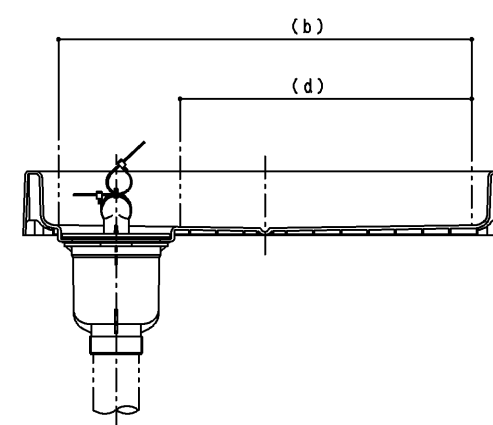
断面B-B
