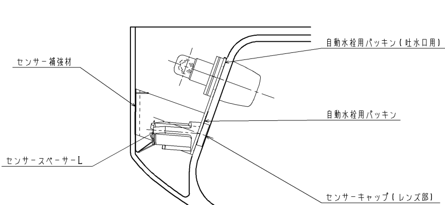
A部断面詳細図 (S=1:2)
