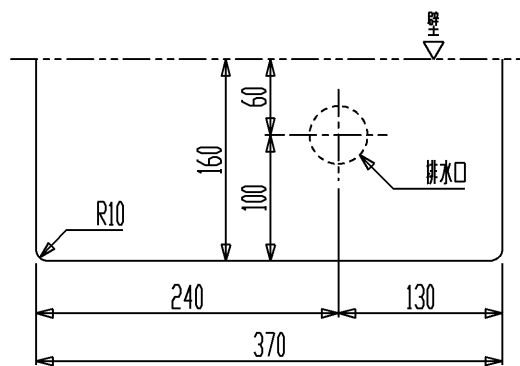
カウンター切込寸法 ※壁に寄せて設置する場合
