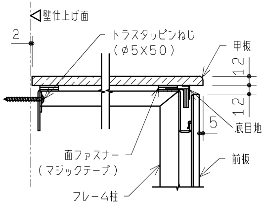
甲板部納まり詳細図（S＝1：5）
