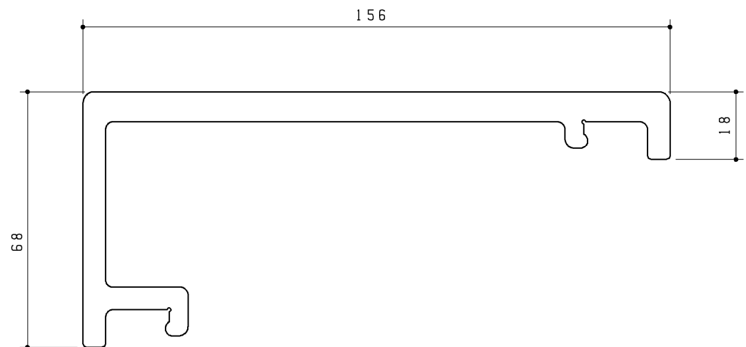
A 視圖 ( S = 1 : 1 )
