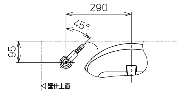
平面图
