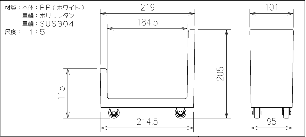
側板組品
