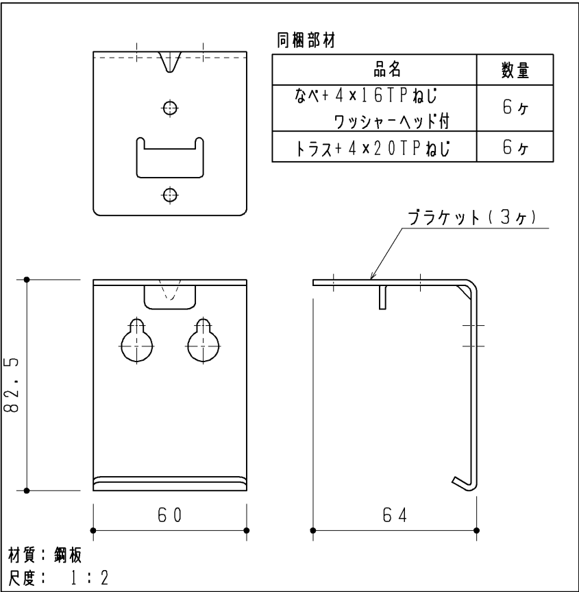
下段ブラケットセット
