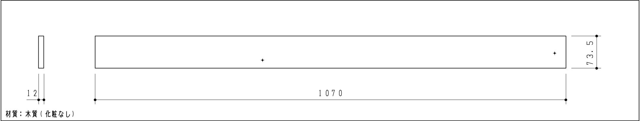
下段補強鉄
