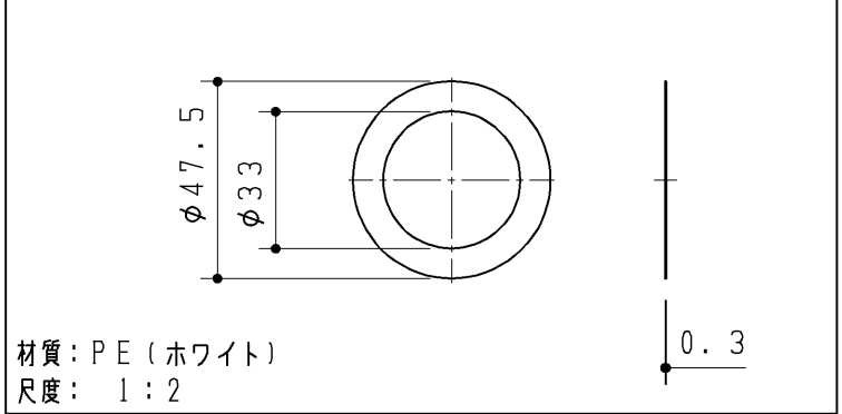
手洗器排水用スリップワッシャー
