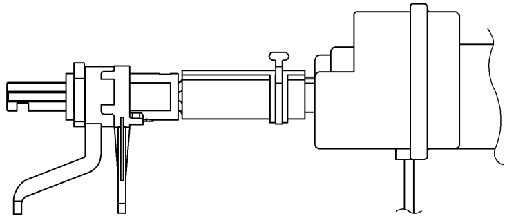
NEW CS(C770系)・NEW CSR(C670系)/寒冷地仕様の場合
