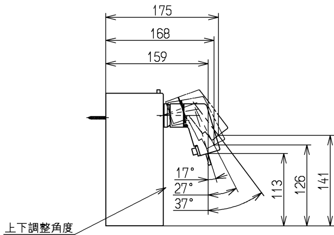
スパウト部(P 視)
