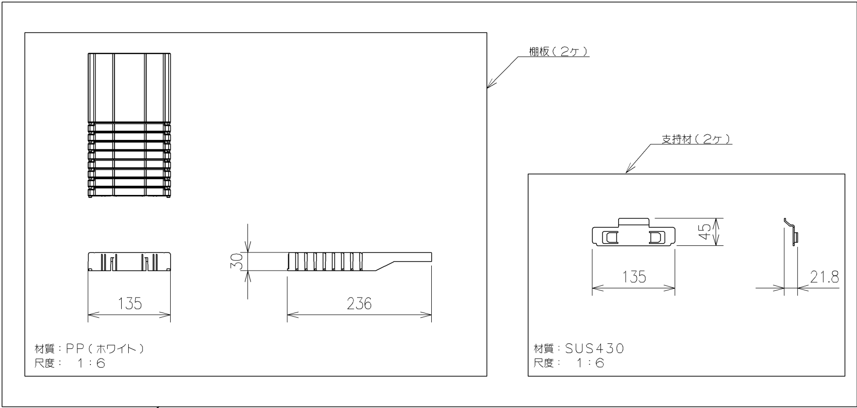
側板組品
