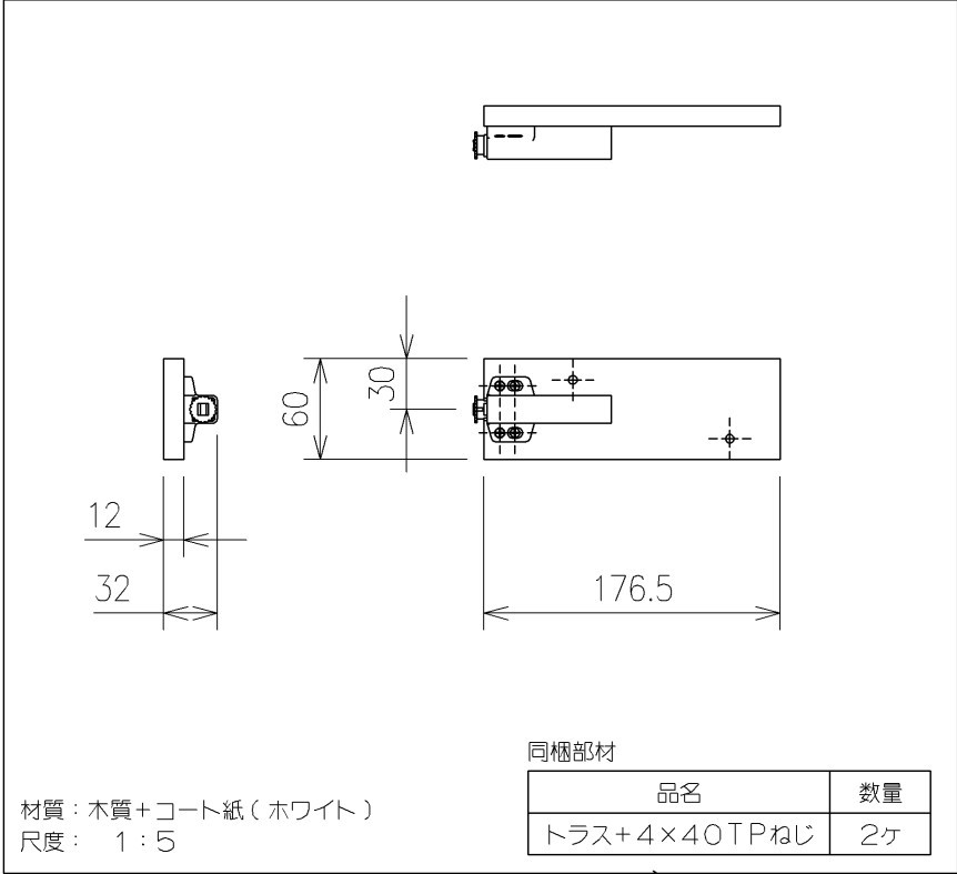
側板組品
